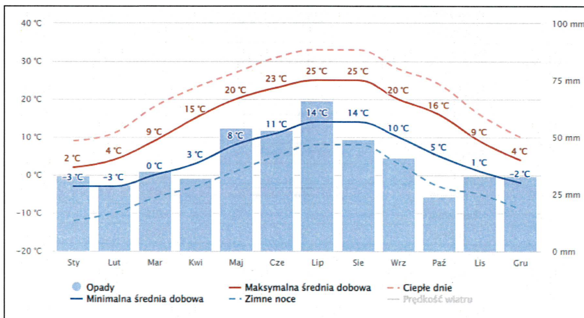
Rysunek 2. Średnie temperatury powietrza oraz opady atmosferyczne na terenie Gminy Siechnice.
