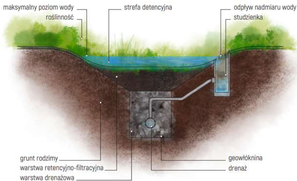
Rysunek 72. Schemat przekroju przez rów bioretencyjny.
