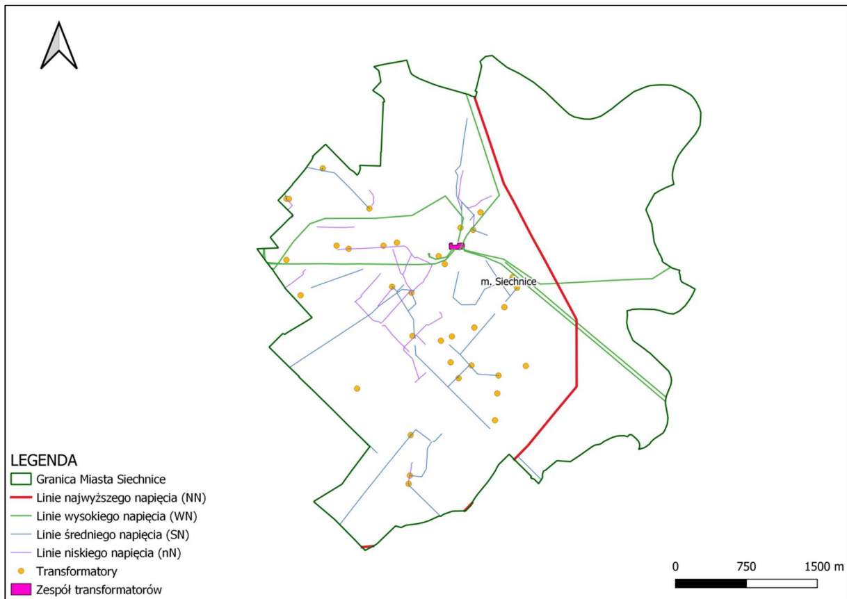
Rysunek 20. Przebieg trasy napowietrznych linii elektroenergetycznych.
