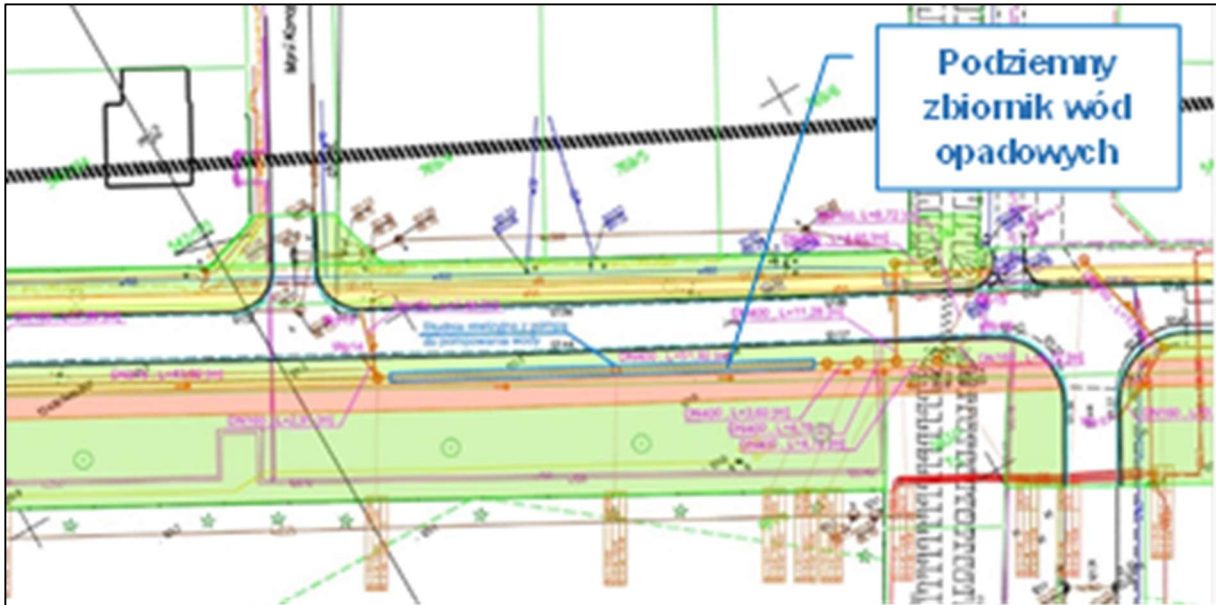
Rysunek 52. Projekt podziemnego zbiornika retencyjnego wód opadowych w pasie zieleni przy ul. Henryka III w Siechnicach.
