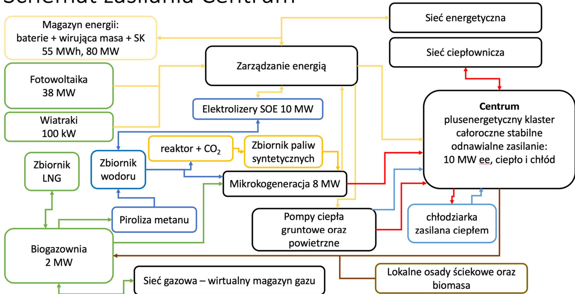
Rysunek 78. Uproszczony schemat systemu zasilania kompleksu EC Czechnica. Źródło: Piotr Pyrka, Zuzanna Czarnecka, Maciej Chorowski, Studium możliwości budowy kompleksu nowych technologii energetycznych w obiektach Elektrociepłowni Czechnica, Politechnika Wroclawska
