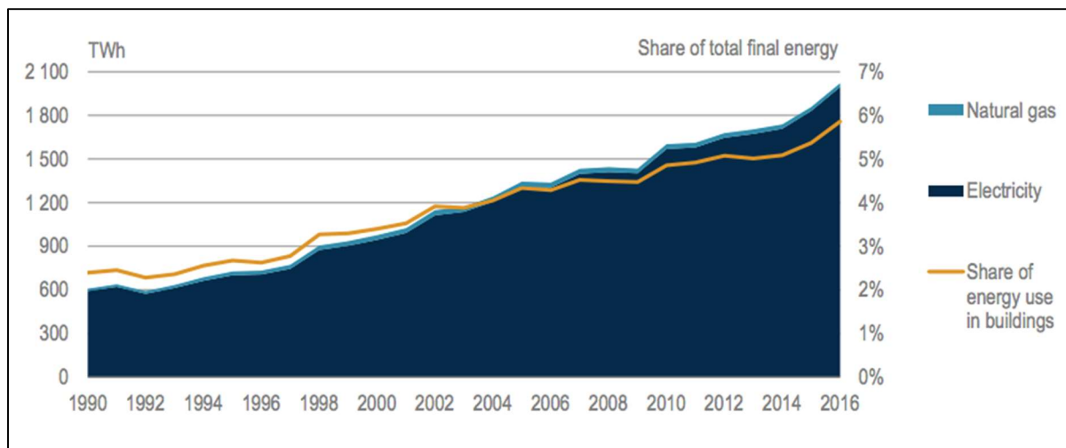
Rysunek 63. Światowe zużycie energii na chłodzenie przestrzeni w budynkach (IEA)
