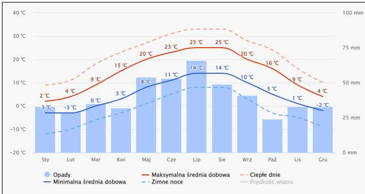
Rysunek 36. Średnie temperatury powietrza oraz opady atmosferyczne na terenie Miasta Siechnice.
