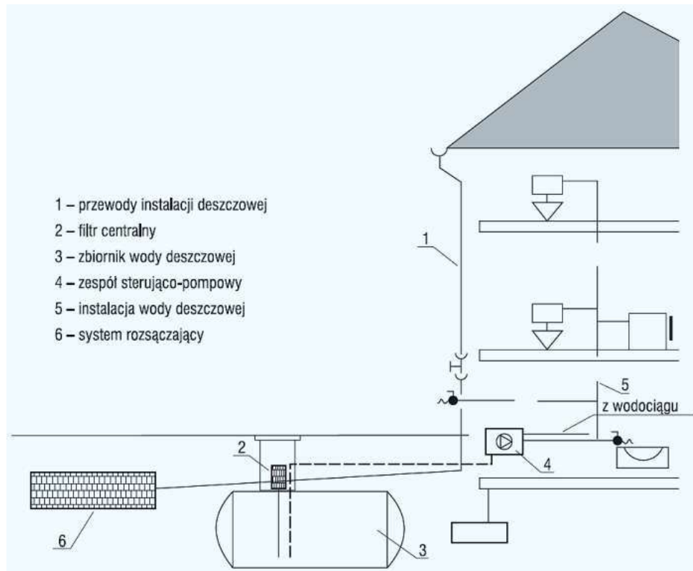
Rysunek 74. Schemat instalacji do wykorzystania wody deszczowej
