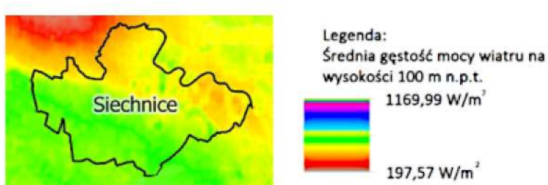
Rysunek 76. Średnia gęstość energii wiatru na wysokości 100 m.
