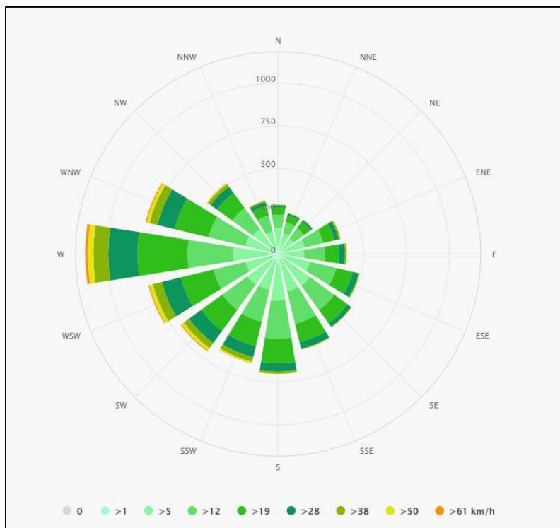
Rysunek 37. Róża wiatrów na terenie Miasta Siechnice.
