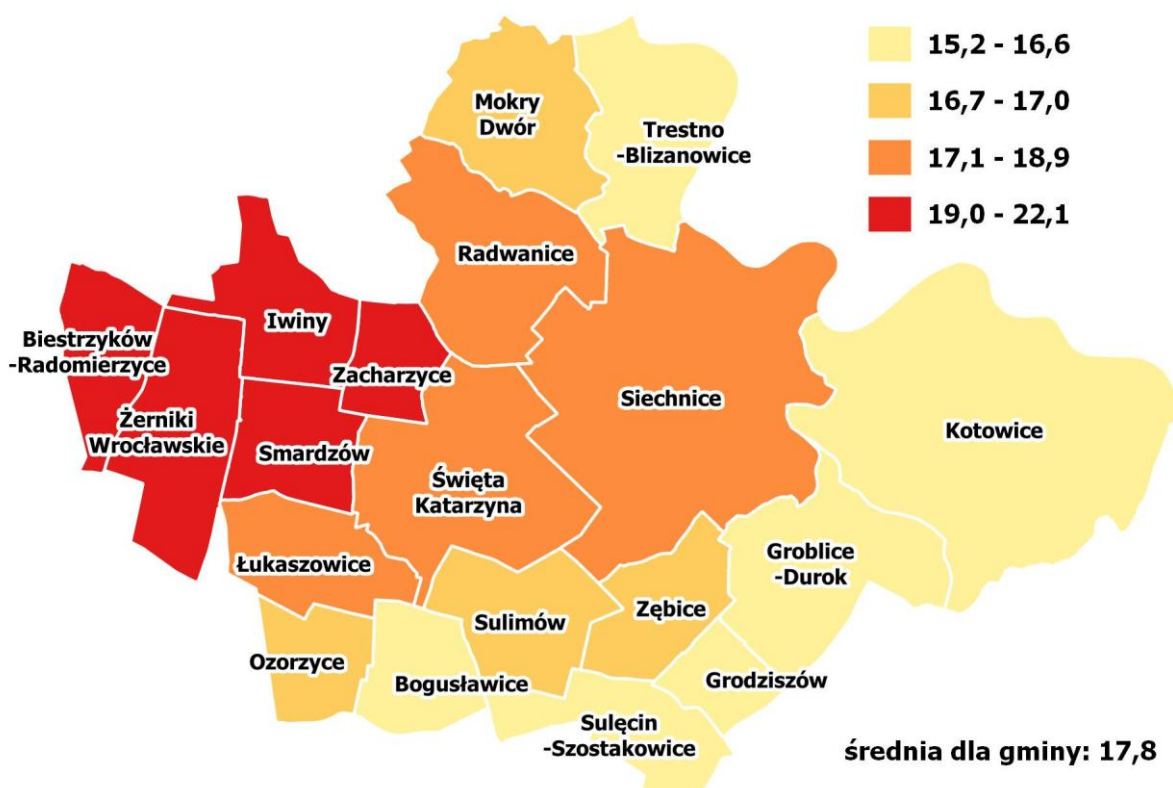
Grafika 20 Średnie roczne stężenie pyłu zawieszonego PM 2,5
